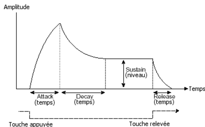
L'enveloppe ADSR
