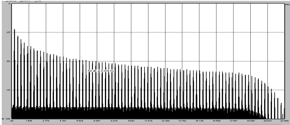
Spectre de réponse fréquentielle du PROPHET V intégrant la technologie TAE
