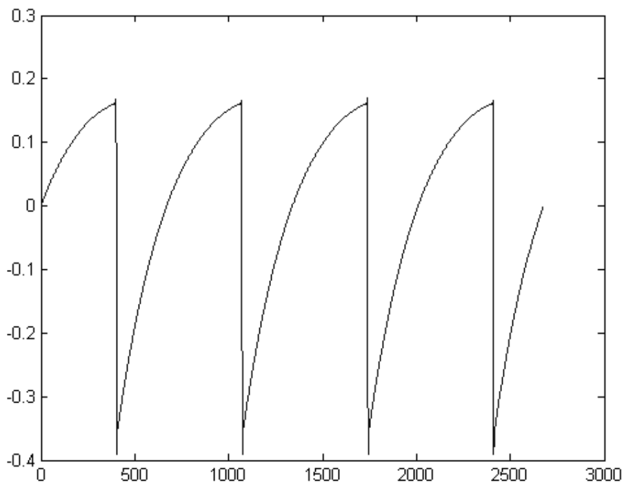
Représentation temporelle de la forme d'onde « dent de scie » du PROPHET V reproduite par TAE
