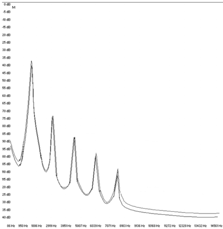
Similitude des courbes de réponse des filtres passe-bas 24 dB du PROPHET 5 et du PROPHET V
