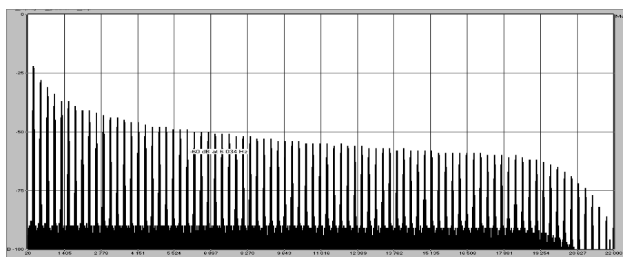
TAE®によって生成されたモーグ・モジュラー V2 のオシレーターによる周波数スペクトラム
