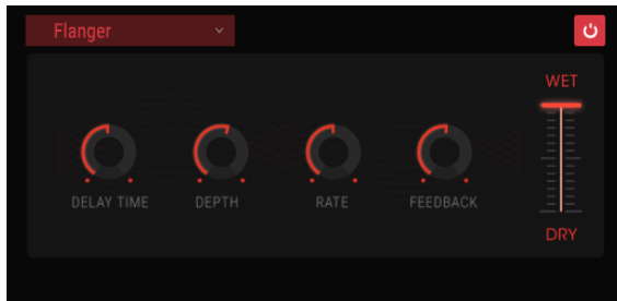
Der Flanger-Effekt
