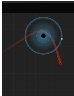
Maximale Gravitationsenergie
