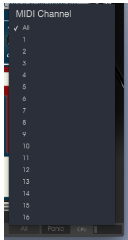
MIDI-Kanaleinstellungen
