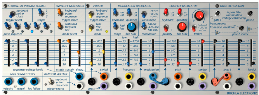
Oktavsprünge
