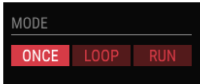
Die Gravity-Mode-Optionen
