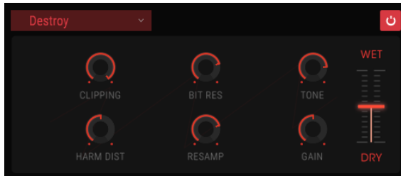
Der Destroy-Effekt
