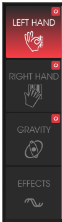
Die Bereichs-Menütaster
