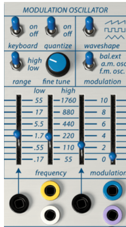
Der Modulationsoszillator
