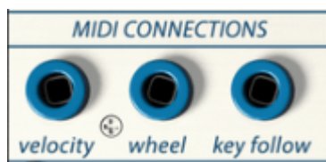
Der MIDI-Anschluss-Bereich
