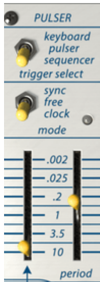
Der Pulser
