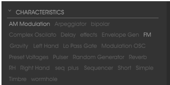
Eingeklapptes Tag-Fenster
