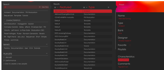
Die Preset-Browser-Schaltfläche
